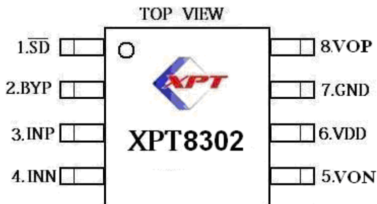
XPT8302 MSOP8、ESOP、SOP封装的管脚分布图
