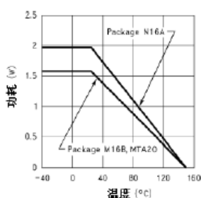
功率下降曲线
