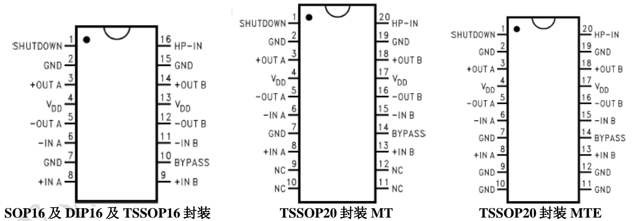
图2 几种封装的管脚示意图
