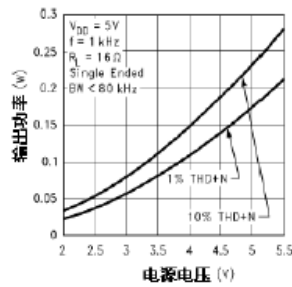
输出功率 vs 电源电压
