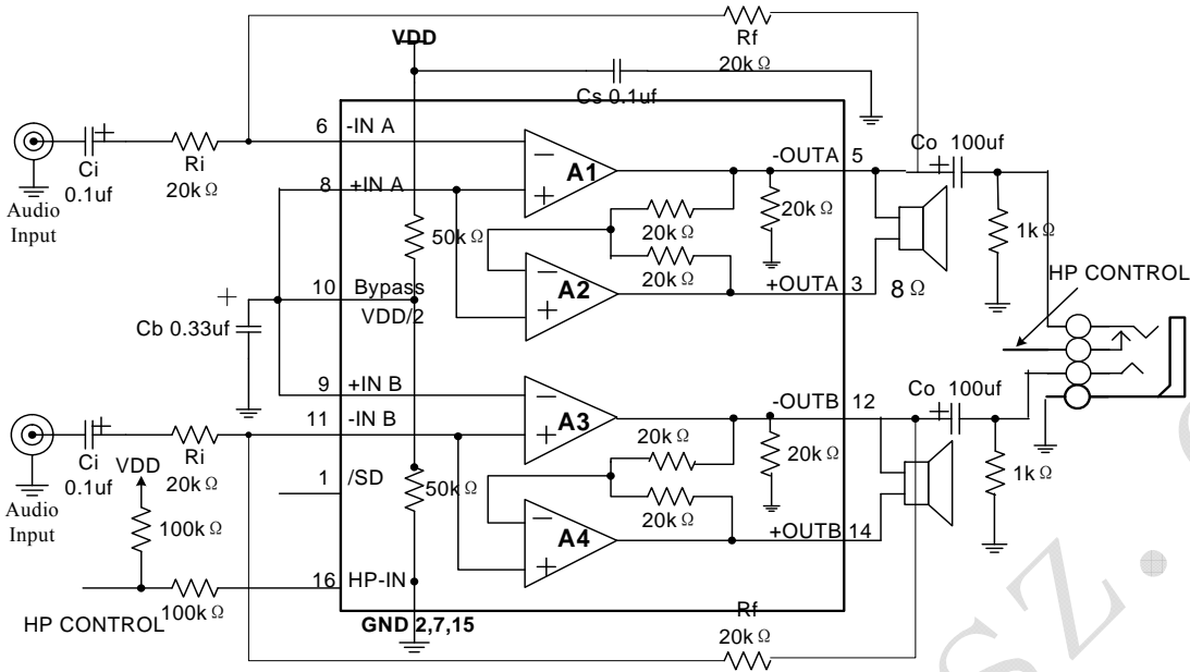
图1 XPT4863 典型应用电路
