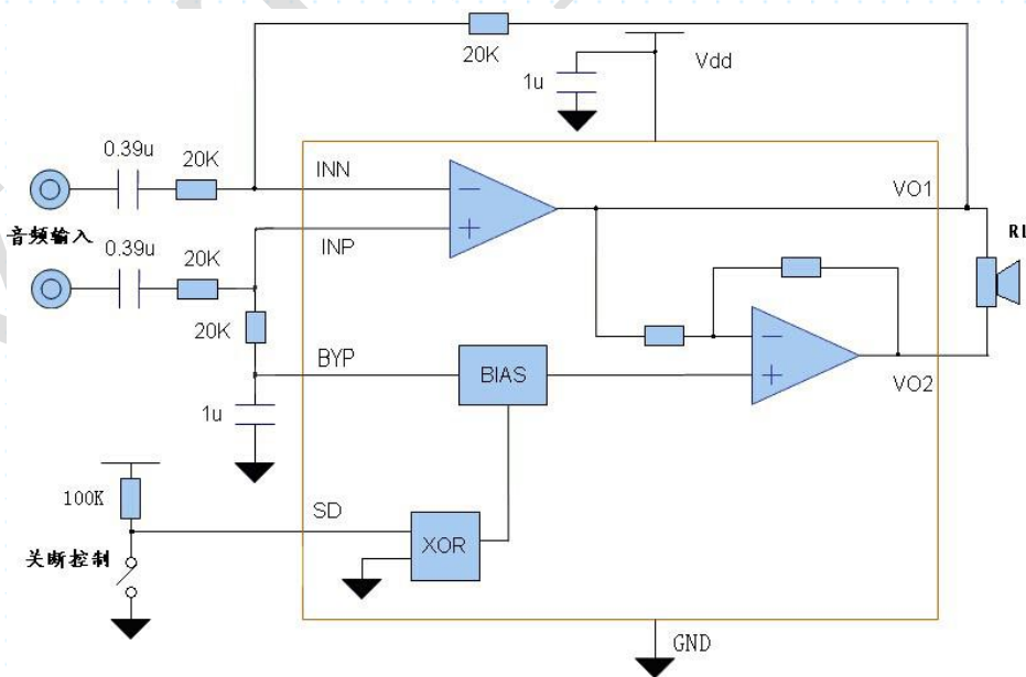
差分输入模式工作电路结构图
